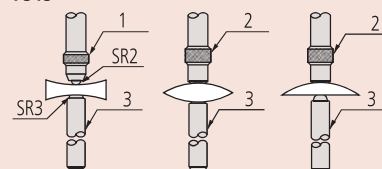
Konkávní čočka Konvexní čočka Plosko-konvexní čočka 1: Kuličkový dotek; 2: Plochý dotek; 3: Pevný dotek
